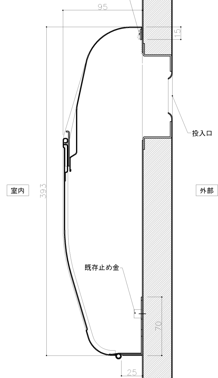
標準納まり図
