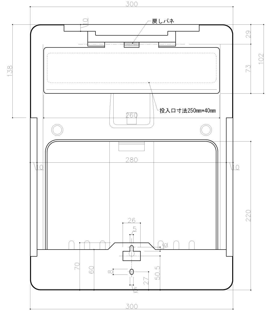
ドア側よりの視図(裏側)
