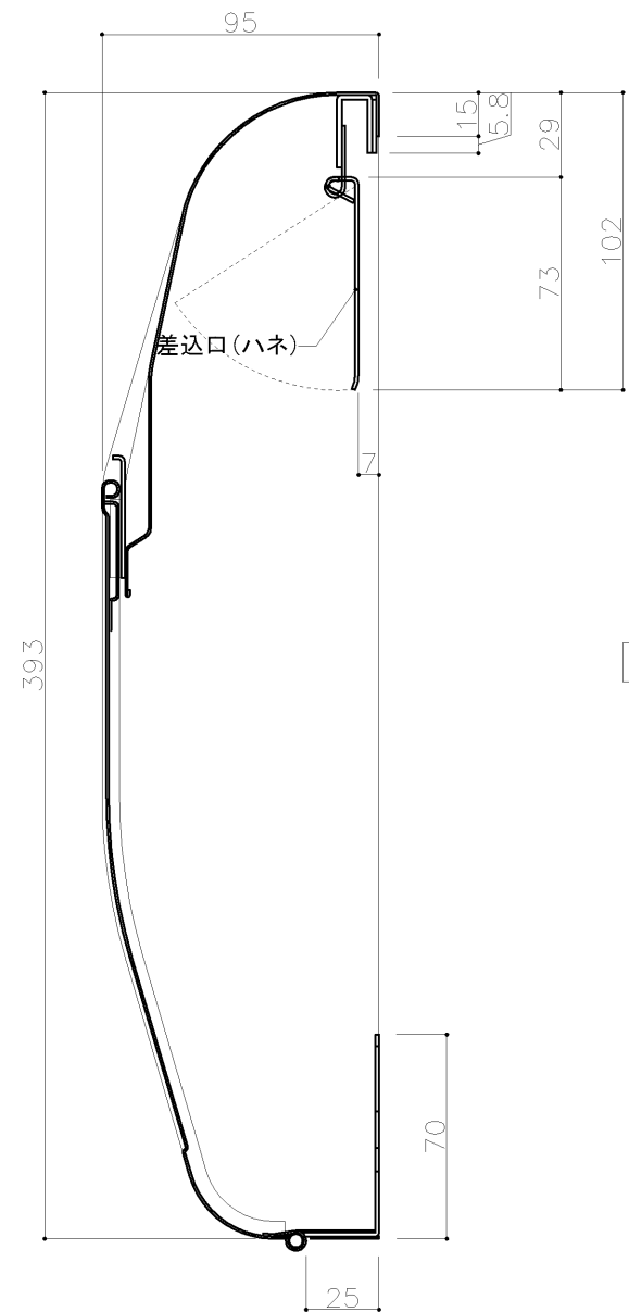
縦断面図
