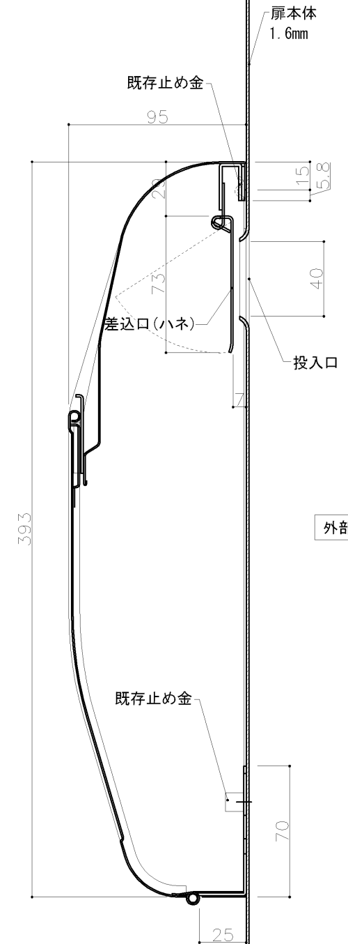
標準納まり図
