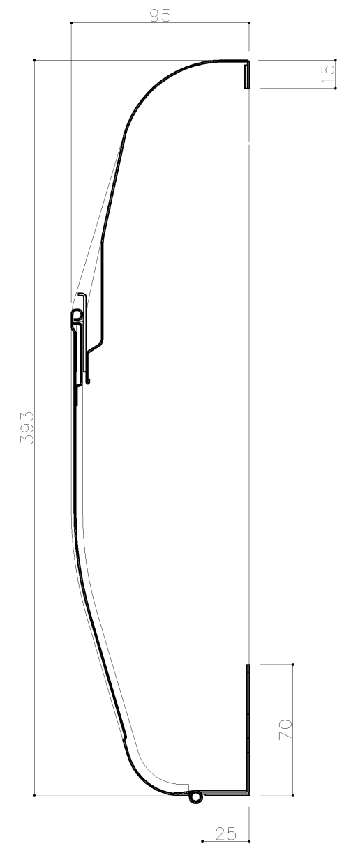
縦断面図
