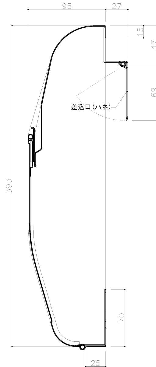
縦断面図
