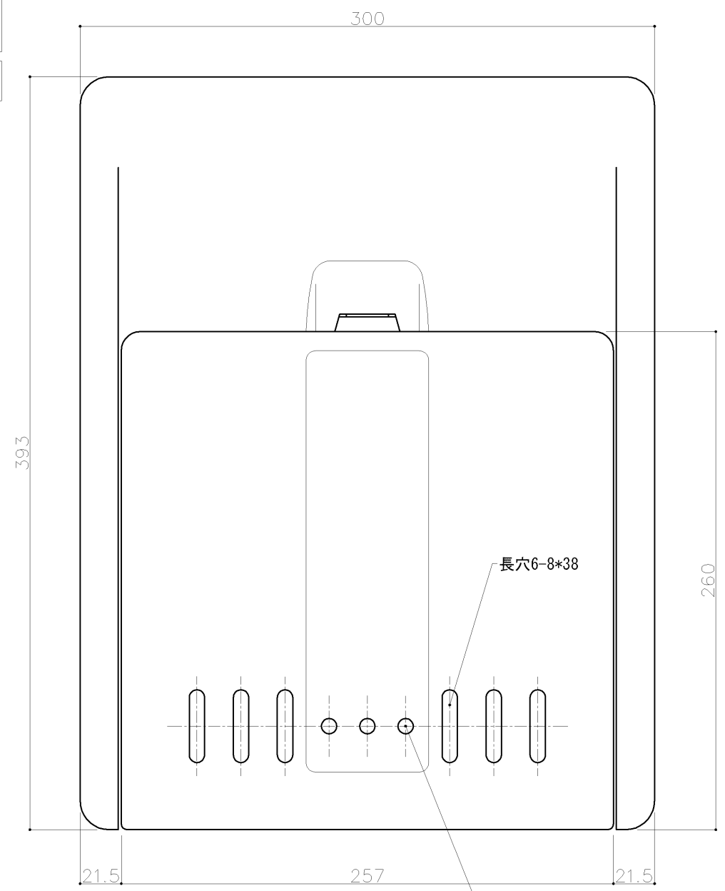
部屋内よりの視図
