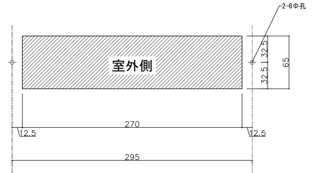
※室外側取付加工図
