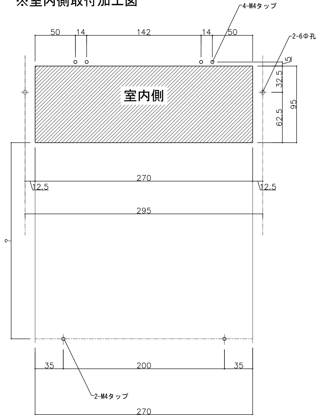
※室内側取付加工図
