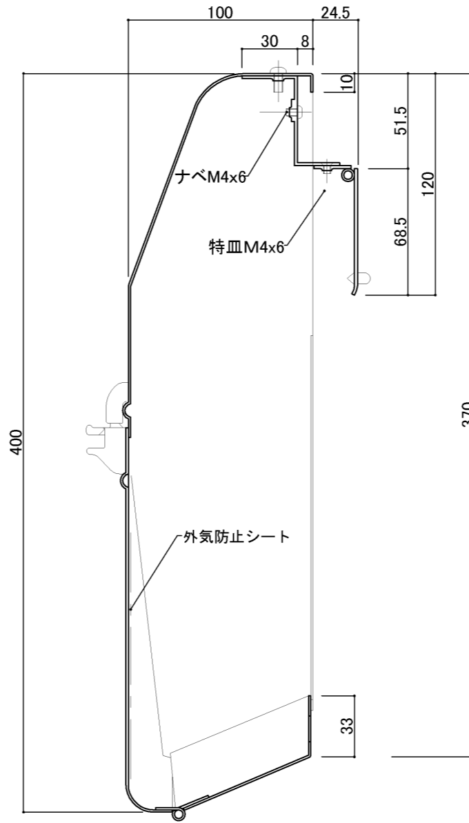
縦断面図
