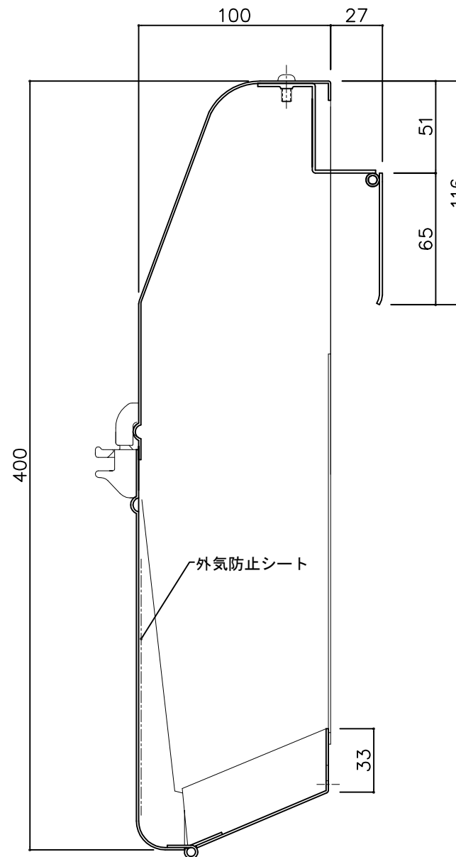
縦断面図
