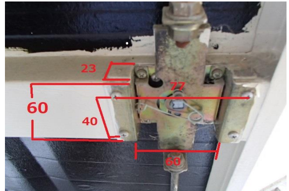
ハンドル裏面・寸法
